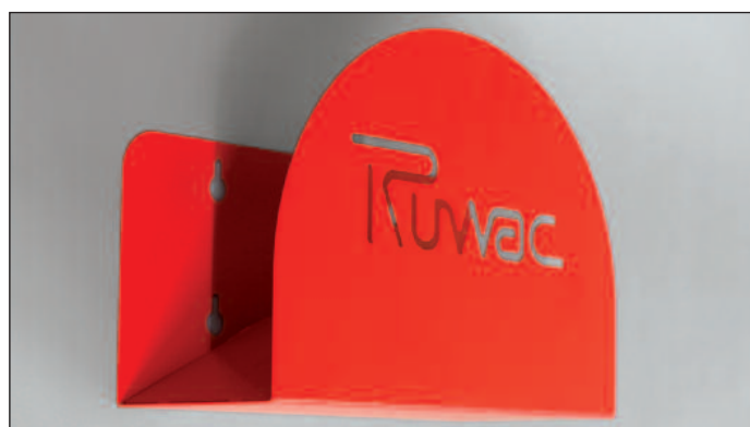
Tömlőtartó, acéllemez, porszórt, piros Falra szerelhető Ho - 330 mm, Szé - 123 mm, Ma - 238 mm rögzítőanyagokkal együtt Cikkszám: 12080
