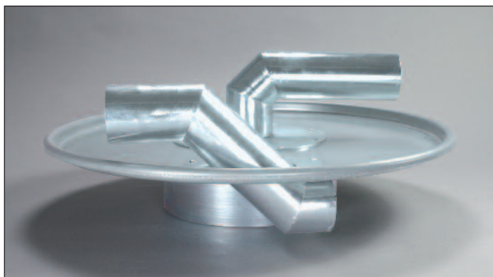
Elő leválasztó fedél, nemesacél, elő leválasztó tartályhoz
