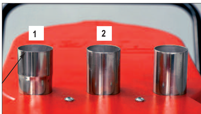
Tartozéktartó, nemesacél, szerelés a hangtompítófedélre Magasság: 65 mm, tartozékhoz 50 mm Ø 1. Belsőátmérő 50 mm - cikkszám: 57121 2. Külsőátmérő 50 mm - cikkszám: 54401
