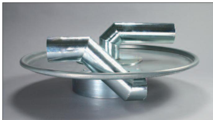
Elő leválasztó fedél, horganyzott acél, elő leválasztó tartályhoz
